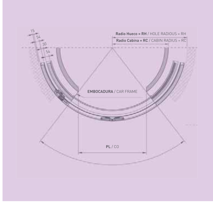
Puerta circular sin marco. Circular door without frame.
