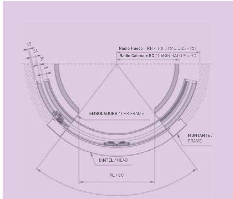
Puerta circular con marco. Circular door with frame.
