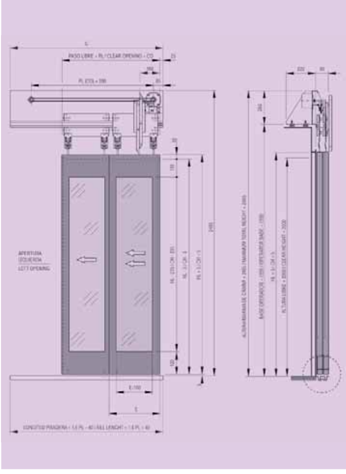
Puerta gran mirilla. Door big vision panel.
